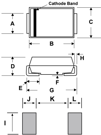
DO-214AA (SMB-Bend)
